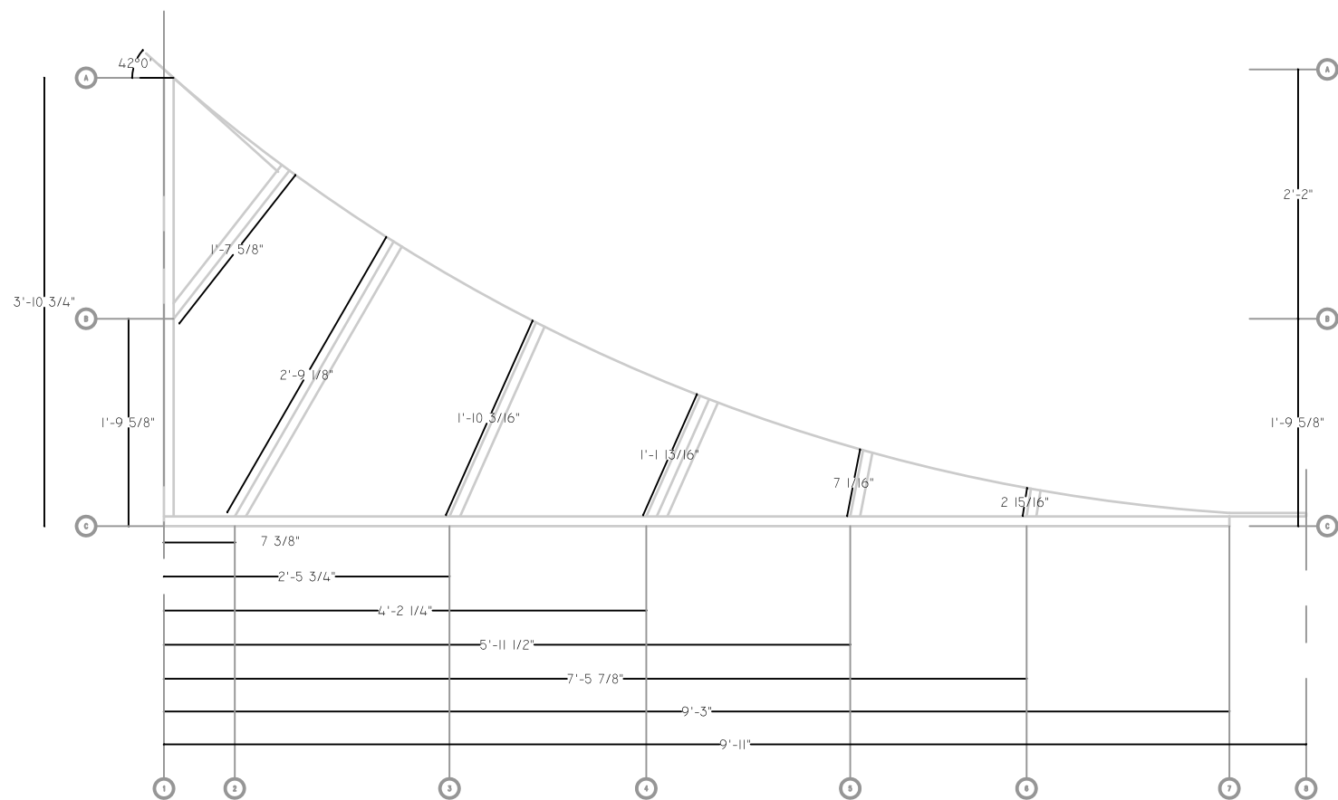
2 RAMP DIMENSIONAL DATA SCALE: NONE
